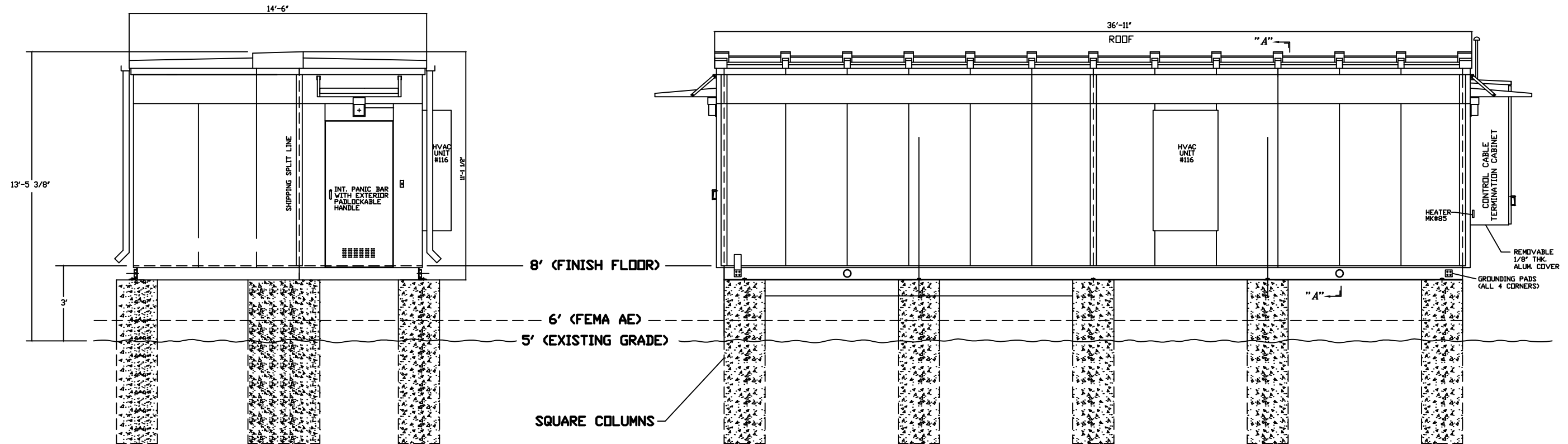
END ELEVATION
