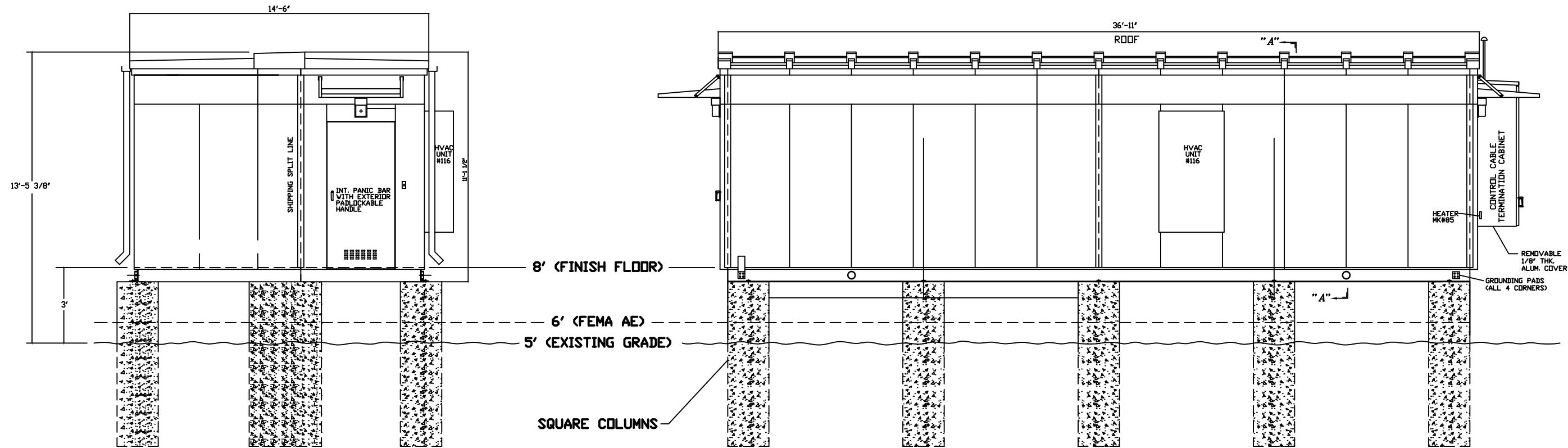
END ELEVATION
