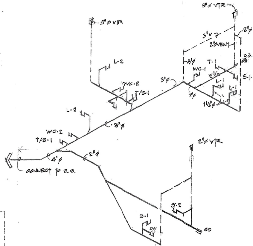
PLUMBING DIAGRAM N.T.S.
