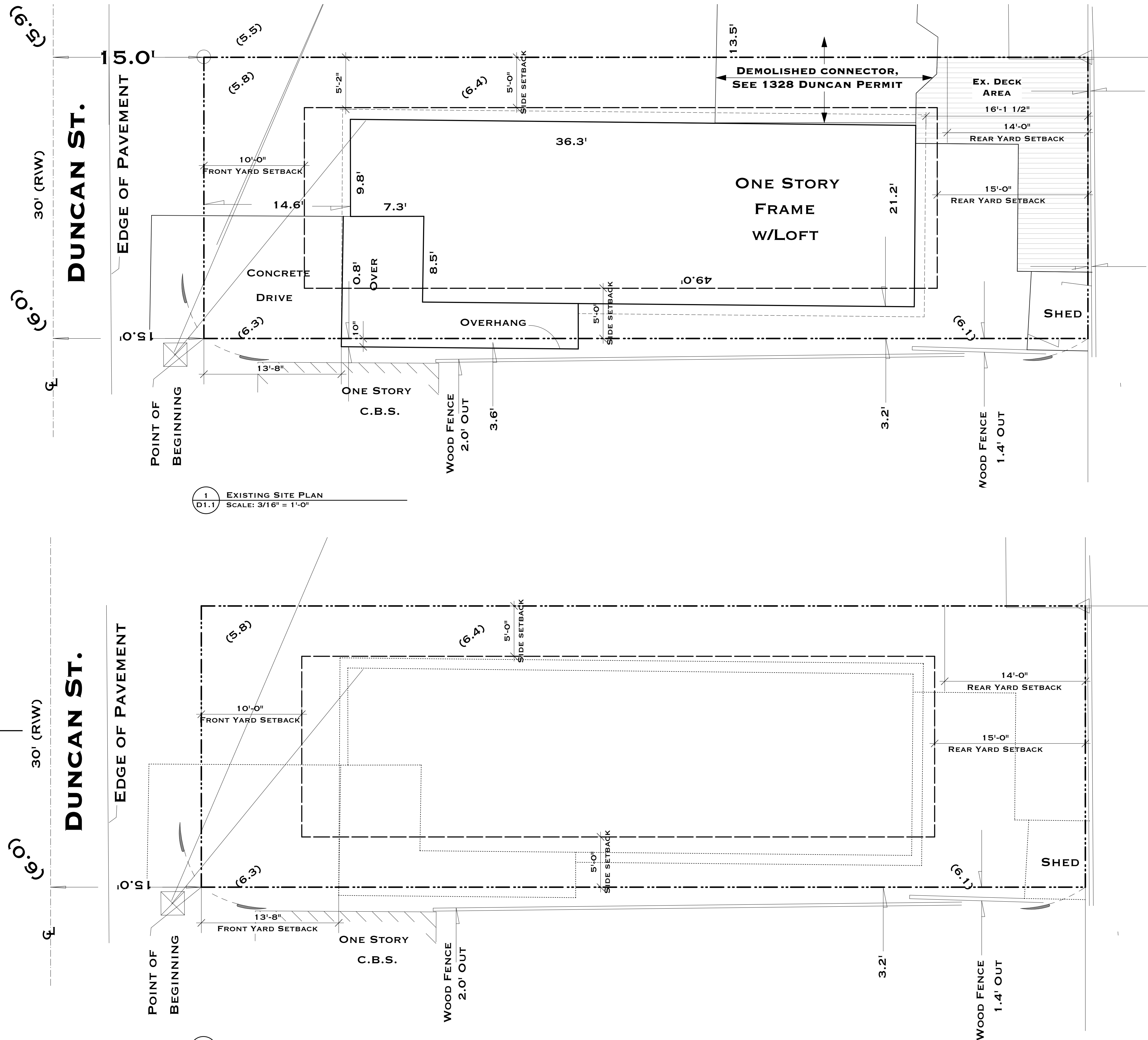
2 DEMOLITION SITE PLAN D1.1 SCALE: 3/16" = 1'-0"
