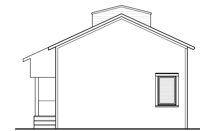
5 EX. ELEVATION - REAR D1.1 SCALE: 1/8" = 1'-0"
