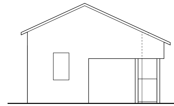
3 EX. ELEVATION - DUNCAN STREET D1.1 SCALE: 1/8" = 1'-0"
