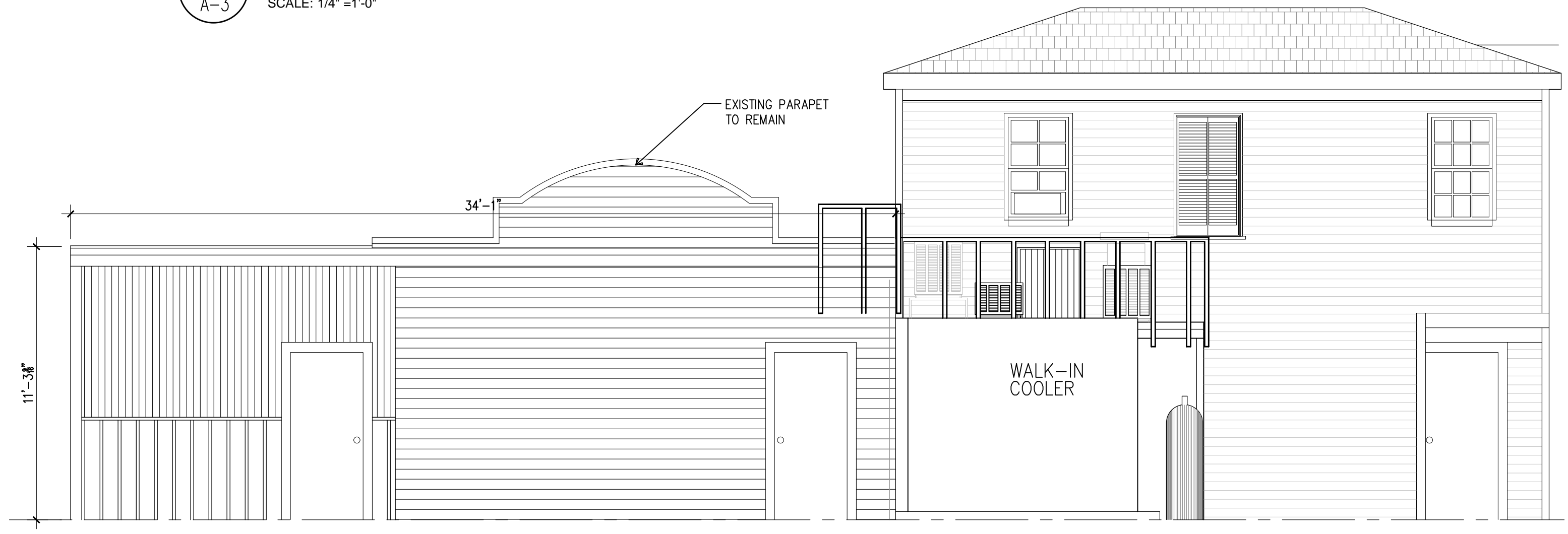
3 EXISTING REAR ELEVATION A-3 SCALE: 1/4" = 1'-0"
