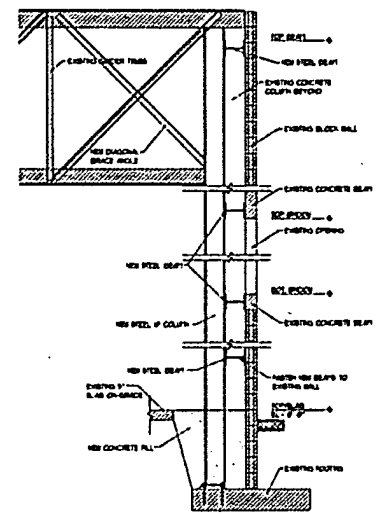
NEW STEEL FRAME 1.1.1.14
