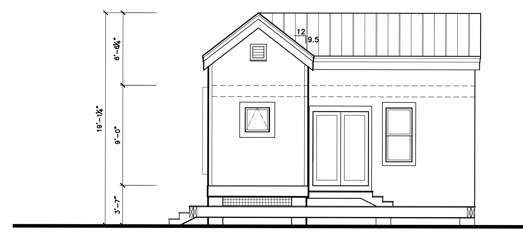
5 INNER ELEVATION A-3 SCALE: 3/16"=1'-0"
