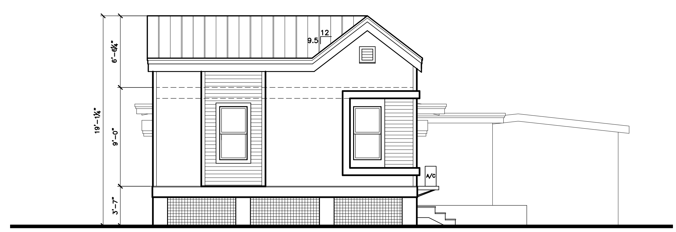
3 REAR ELEVATION A-3 SCALE: 3/16"=1'-0"
