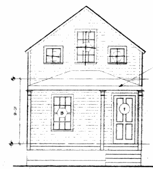
FRONT (LANE) ELEVATION
