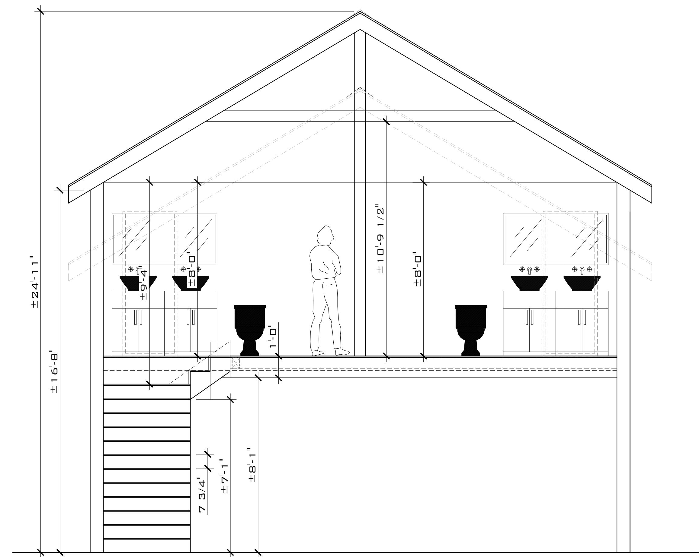
SECTION 1-2 SCALE: 3/8" = 1'-0"
