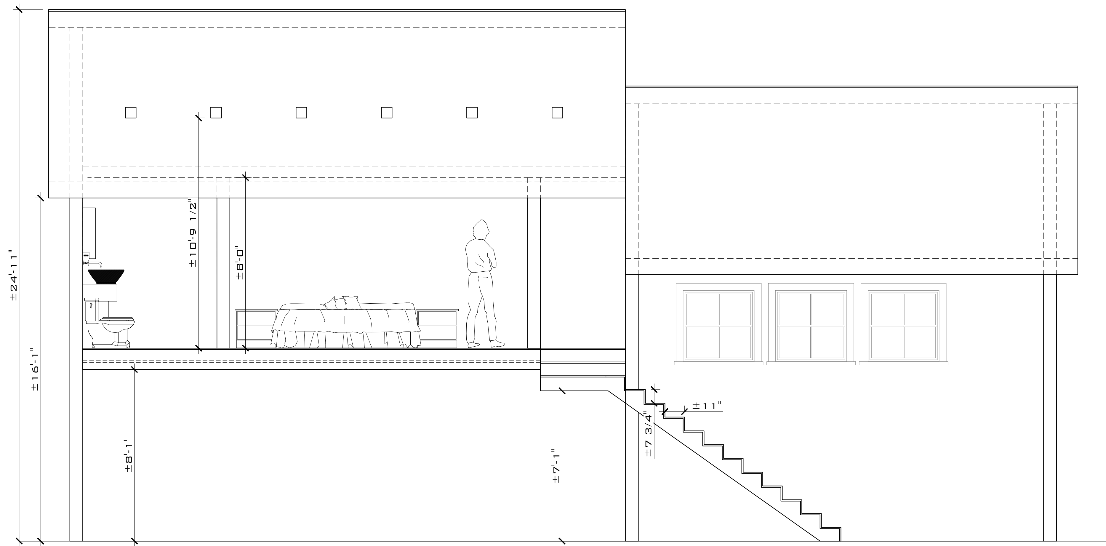
SECTION 1-3 SCALE: 3/8" = 1'-0"
