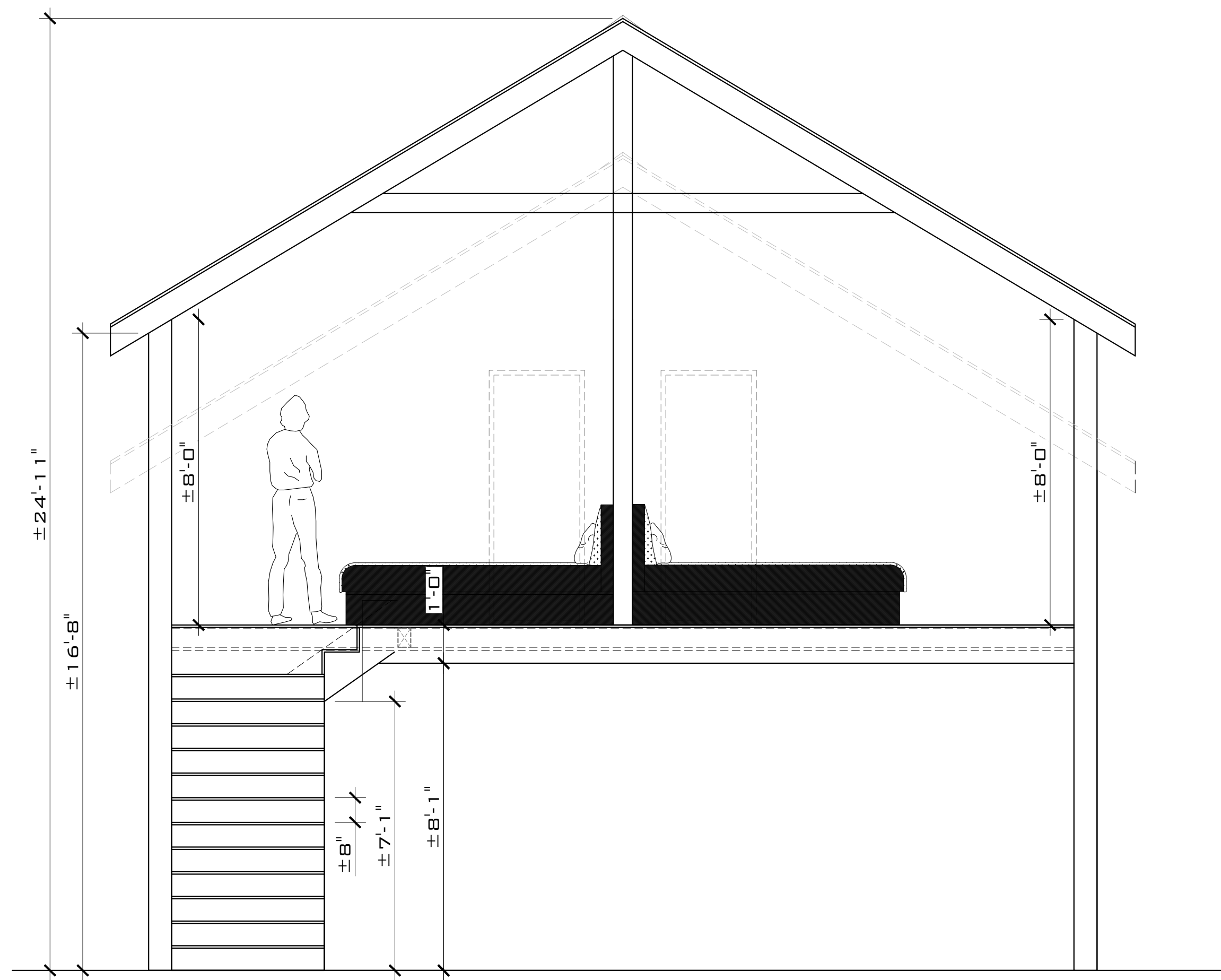
SECTION 1-1 SCALE: 3/8" = 1'-0"
