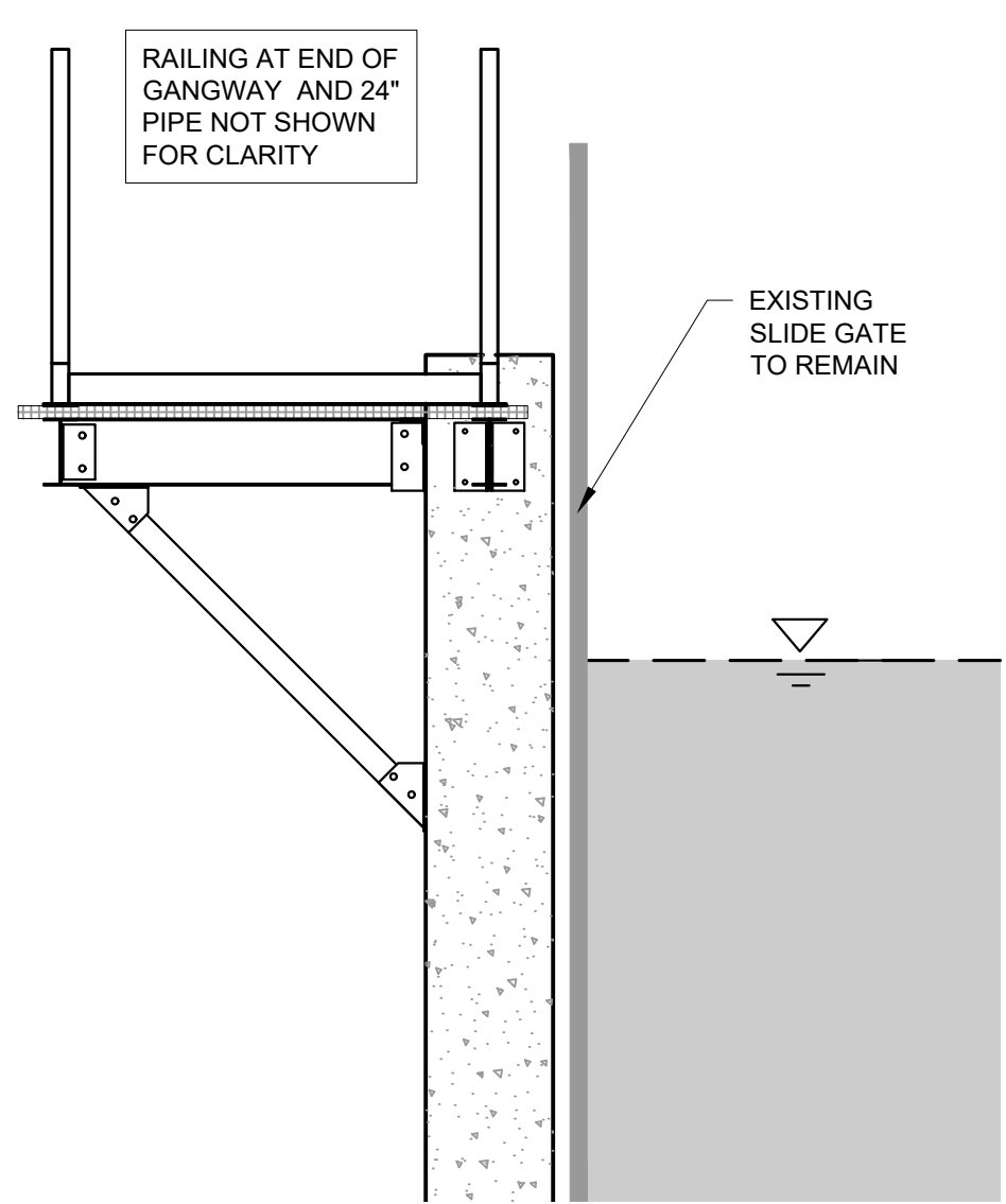
B SECTION - GANGWAY 1 S-1 EXISTING SCALE: 1/2"=1'-0"
