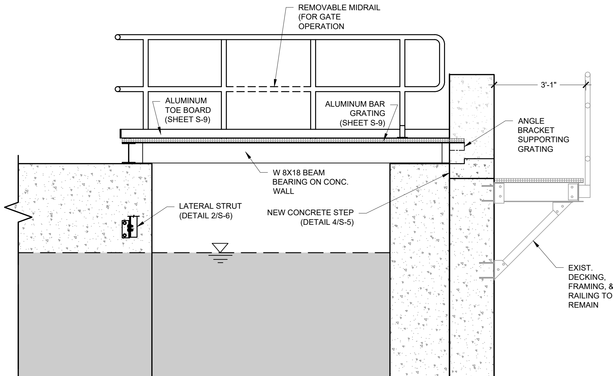
A SECTION - GANGWAY 2
