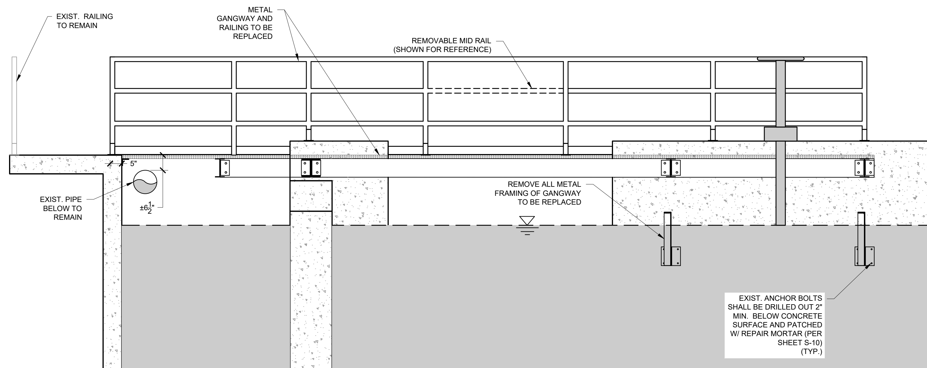
SECTION - GANGWAY 4
