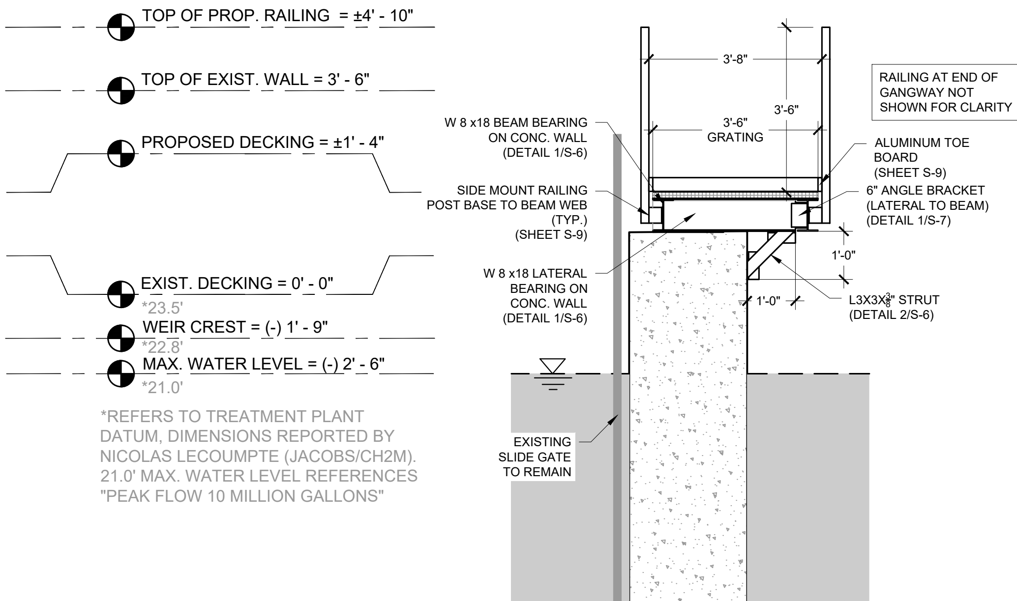
B S-7 SECTION - GANGWAY 3
