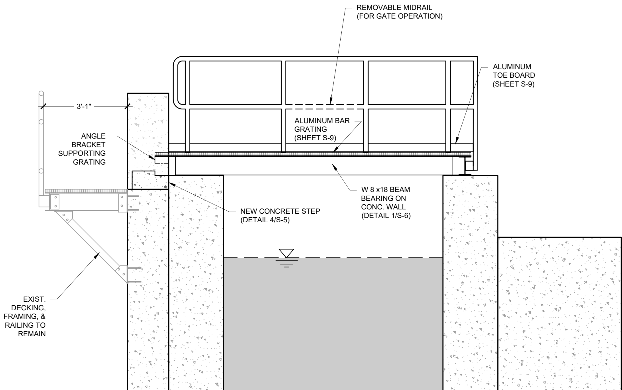
SECTION - GANGWAY 3
