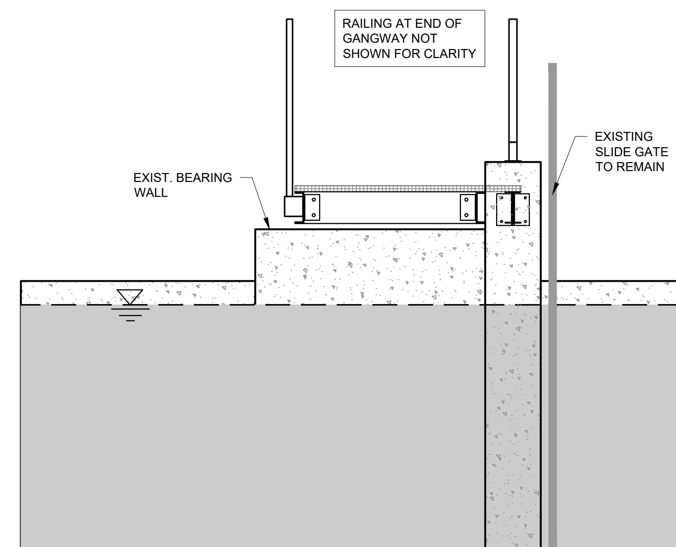
SECTION - GANGWAY 4
