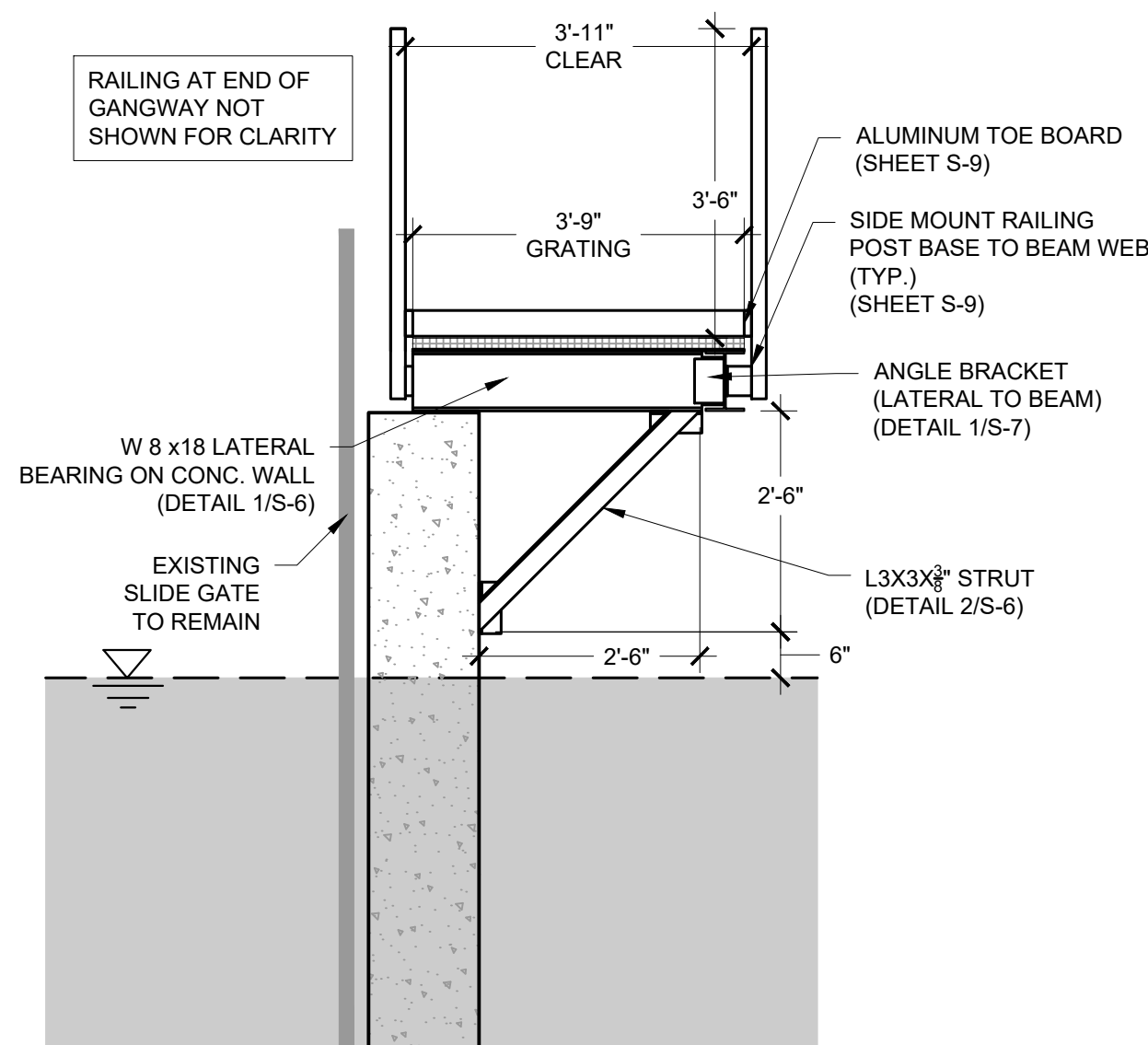
B SECTION - GANGWAY 2
